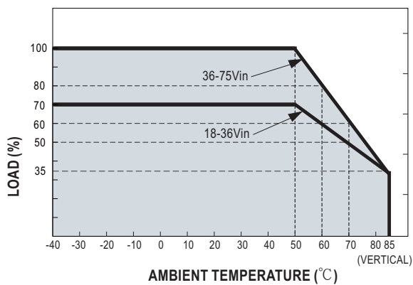
DDR-60L-5V
